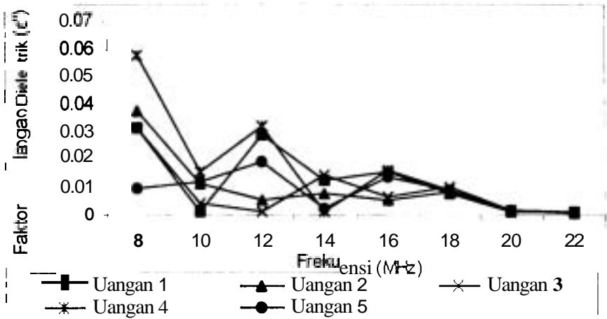
Gambar 8. Grafik pengaruh frekuensi terhadap nilai faktor kehilangan dielektrik ( \epsilon'' ) lada (kadar air 13,82 % bb) nilai Q dibaca pada arus bolak-balik (AC)
