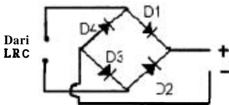
Gambar 4. Rangkaian Jembatan dioda untuk mengubah arus bolak-balik (AC) ke arus searah (DC)
