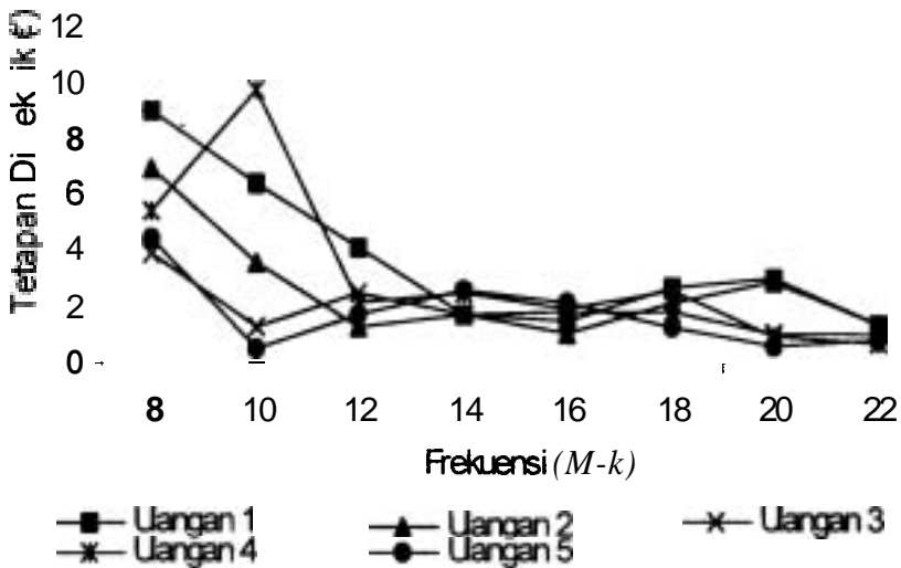
Gambar 9. Grafik pengaruh frekuensi terhadap tetapan dielektrik ( \epsilon' ) lada (kadar air 13.8 % bb) nilai Q dibaca pada arus searah (DC)
