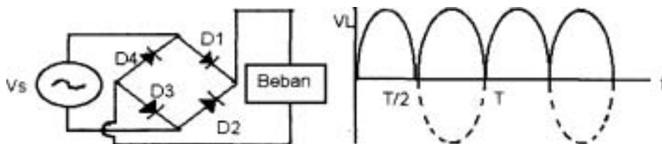
Gambar 3. Rangkaian penyearah gelombang penuh dengan jembatan dioda ( dioda bridge ) (Zuhal, 1995)
