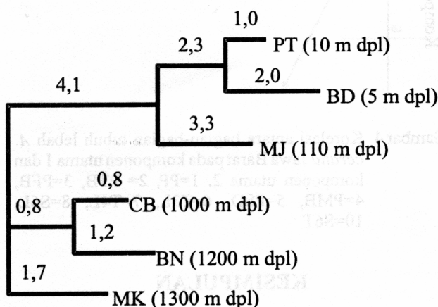
Gambar 2 Dendogram lebah A. cerana di Jawa Barat. Angka-angka pada tiap cabang menunjukkan jarak ketidaksamaan antara ujung cabang dengan nodus atau antara nodus dengan nodus. PT, BD, MJ, CB, BN, dan MK menunjukkan nama lokasi (lihat Tabel 1)
