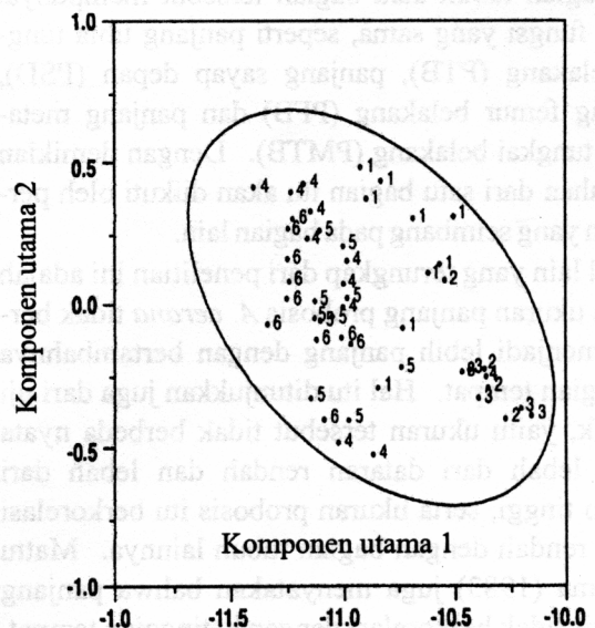
Gambar 3 Plot penyebaran lebah A. cerana Jawa Barat pada komponen utama 1 dan komponen utama 2. Dataran rendah 1=BD, 2=PT, 3= MJ. Dataran tinggi 4=CB, 5=BN, 6=MK
