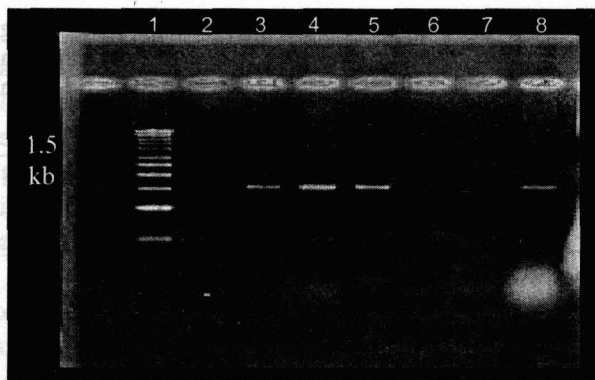
Gambar 1. Hasil amplifikasi DNA virus gemini dengan PCR. Lajur 1: marker 1kb; 2-tanaman sehat sebagai kontrol negatif; 3-hasil penularan pada tanaman cabai rawit; 4-hasil penularan pada tanaman tomat; 5-hasil penularan pada tanaman cabai besar; 6-hasil penularan pada tanaman tomat; 7-hasil penularan pada tanaman tembakau; 8-kontrol positif (klon DNA-pepper leaf curl virus Thailand)
