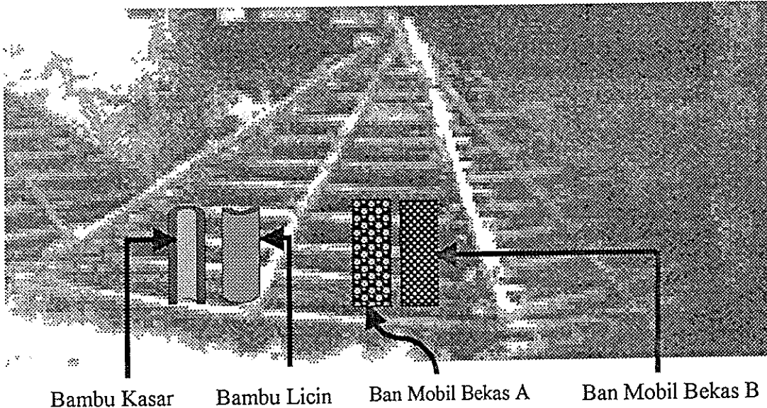
Gambar 4. Potongan bambu dan ban mobil bekas yang diletakkan pada terumbu karang buatan bambu sebagai tempat menempelnya perifiton
