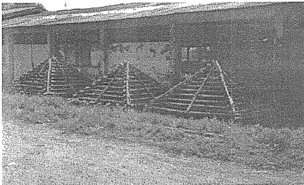
Gambar 2. Struktur modul terumbu karang buatan bambu yang diletakkan pada lokasi penelitian
