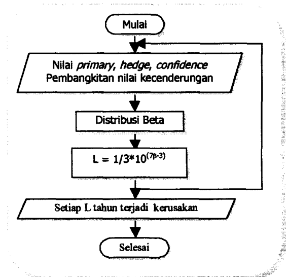
Gambar 5. Diagram alir deskriptif tahun mendatang terjadinya pencemaran produk minuman konsentrat sari buah
