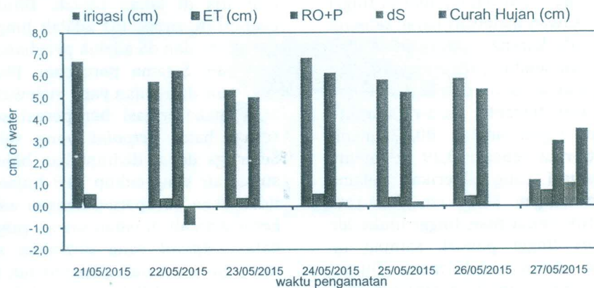
Gambar 11 Akumulasi Komponen Kesenjangan Air pada Percobaan Irigasi Otomatis
