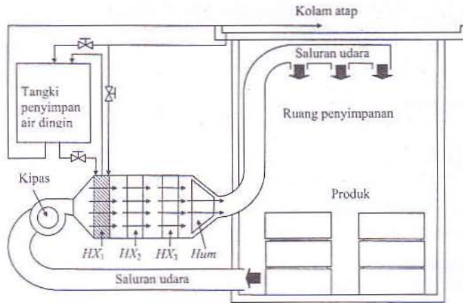
Gambar 1. Skema instalasi penyimpanan dingin di Desa Candikuning Bali.
