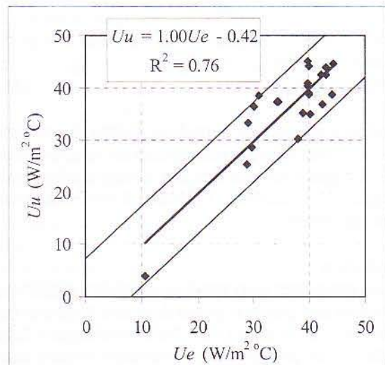
Gambar 7. Diagram serak dari hubungan U_e dengan U_u .
