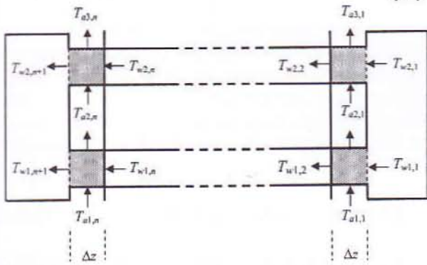
Gambar 3. Penampang alat penukar panas dilihat dari atas.
