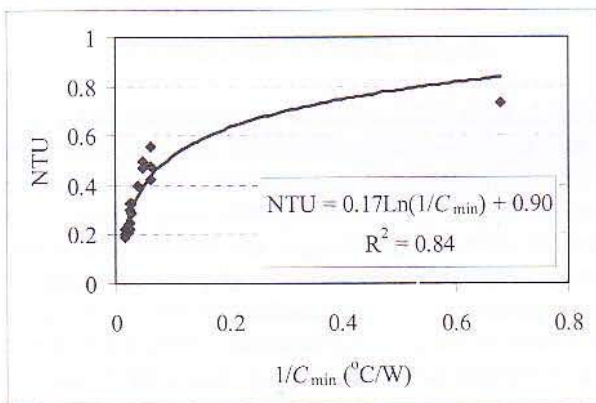
Gambar 5. Pengaruh laju aliran massa air terhadap nilai NTU alat penukar panas.
