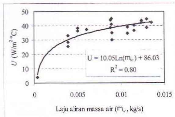
Gambar 4. Pengaruh laju aliran massa air terhadap nilai U alat penukar panas.
