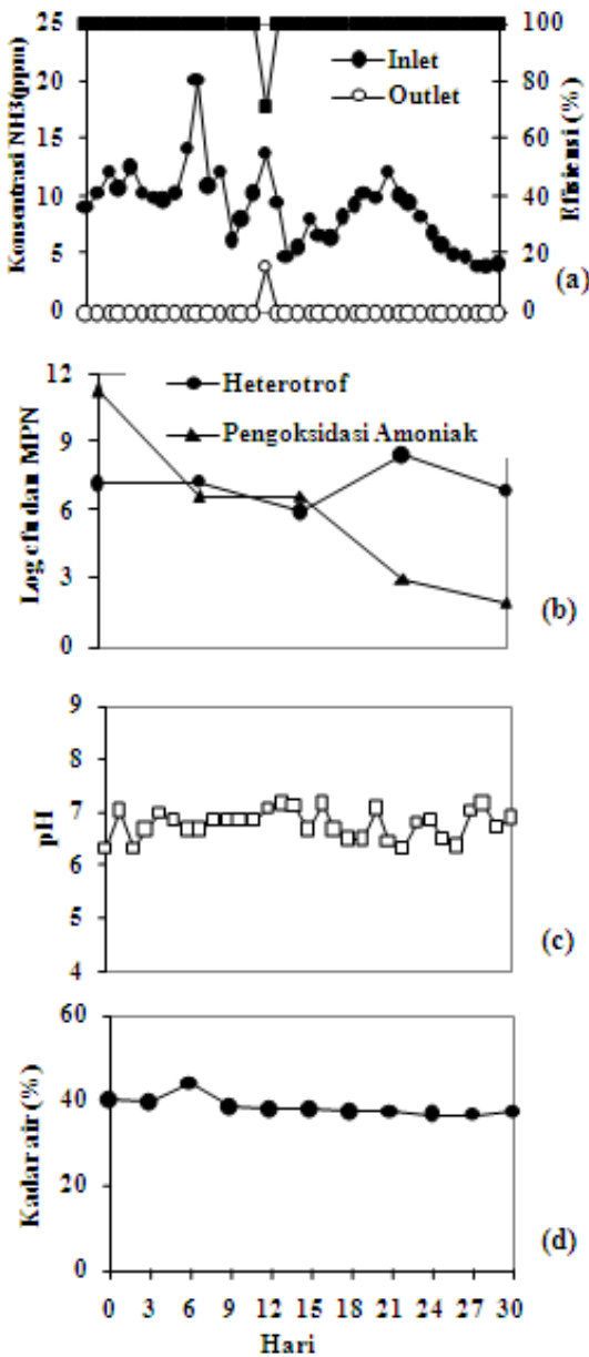
Gambar 4. Kondisi dan kinerja penghilangan amoniak pada biofilter #3 (a) Inlet- outlet, dan efisiensi amoniak (b) populasi bakteri, (c) pH, (d) Kadar air bahan pengisi.
