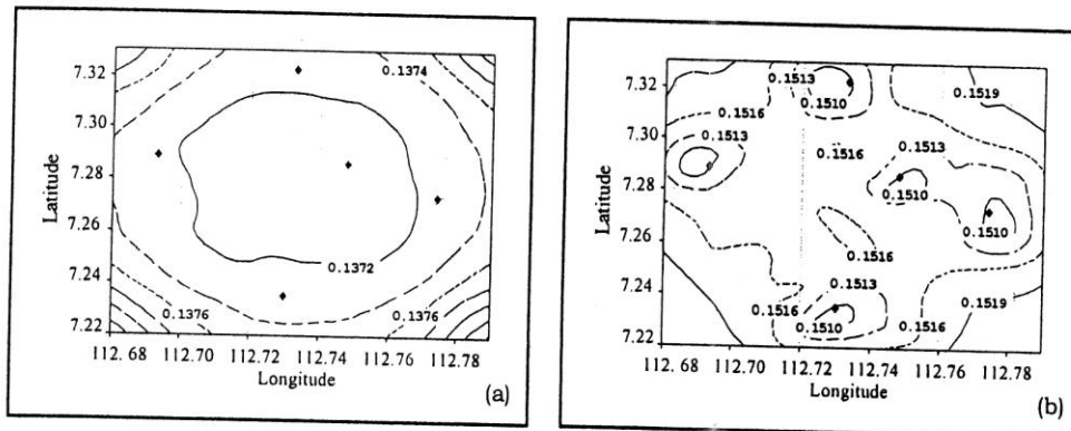
Gambar 1. Pola ragam spatial untuk PM 10 (a) Model-7 dan (b) Model-8
