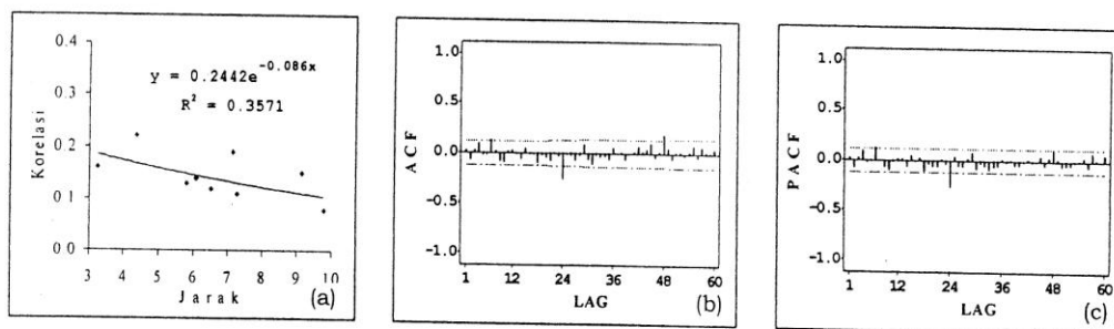
Gambar 2. (a) Plot korelasi spasial, (b) Plot ACF, dan (c) Plot PACF dari galat Model-8
