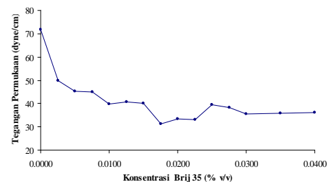
Gambar 2 Tegangan permukaan Brij 35.
