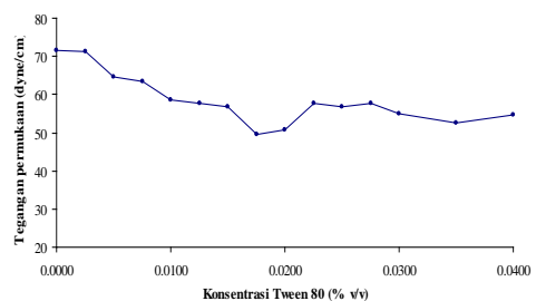
Gambar 1 Tegangan permukaan Tween 80.
