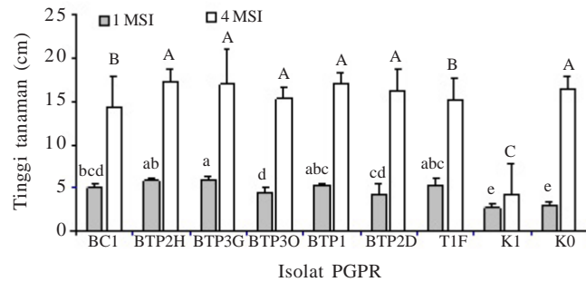
Gambar 2. Rata-rata tinggi tanaman cabai Tit Segitiga (N=5) pada 1 minggu setelah inokulasi (MSI) dan 4 MSI yang diberi perlakuan PGPR dan inokulasi ChiVMV. K1: tanpa PGPR tetapi diinokulasi dengan ChiVMV, K0: kontrol (tanpa PGPR dan tanpa inokulasi ChiVMV). Perbedaan huruf menunjukkan beda nyata berdasarkan DMRT pada taraf nyata 5%.
