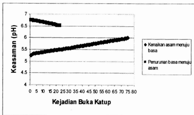
Gambar 2. Grafik keasaman larutan nutrisi dalam rentang set point .
