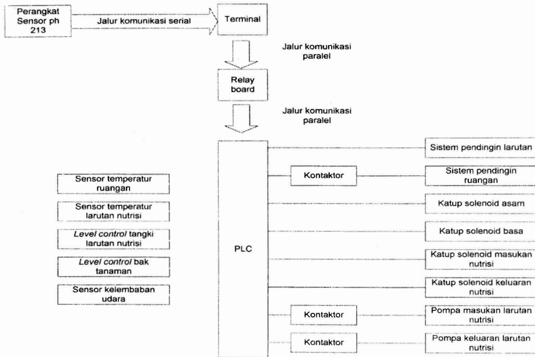
Gambar 1. Diagram blok rancangan fungsional
