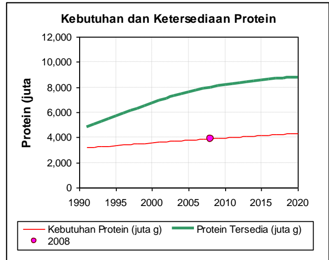
Gambar 13. Proyeksi kebutuhan dan ketersediaan protein di Kabupaten Aceh Selatan tahun 1991-2020
