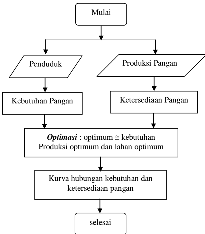
Gambar 1. Diagram optimasi pangan
