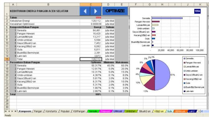
Gambar 2. Optimasi komposisi bahan makanan
