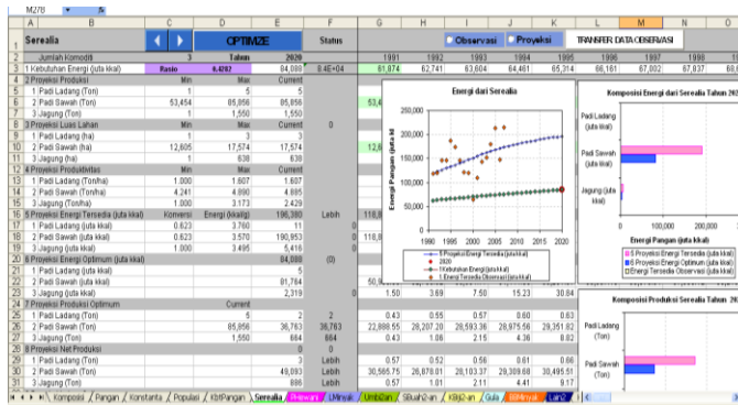
Gambar 3. Optimasi kelompok makanan serealia
