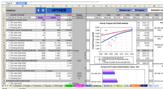
Gambar 5. Optimasi kelompok makanan umbi-umbian
