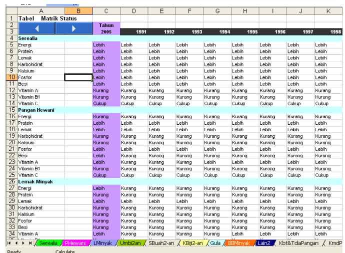
Gambar 6. Status ketersediaan pangan
