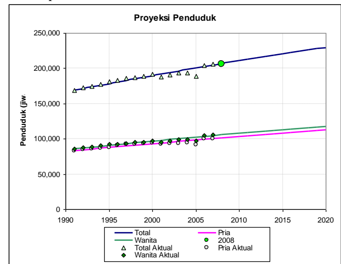
Gambar 7. Proyeksi penduduk Kabupaten Aceh Selatan tahun 1991-2020
