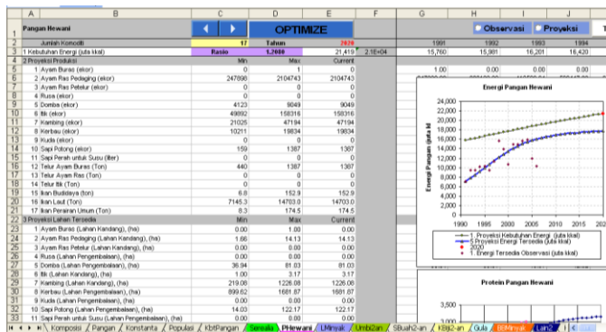
Gambar 4. Optimasi kelompok makanan pangan hewani
