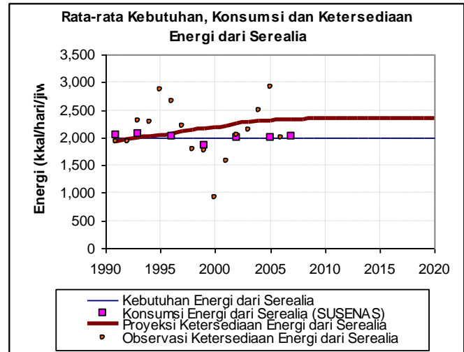
Gambar 10. Rata-rata kebutuhan, konsumsi, dan ketersediaan energi perkapita dari sereal di Kabupaten Aceh Selatan tahun 1991-2020.
