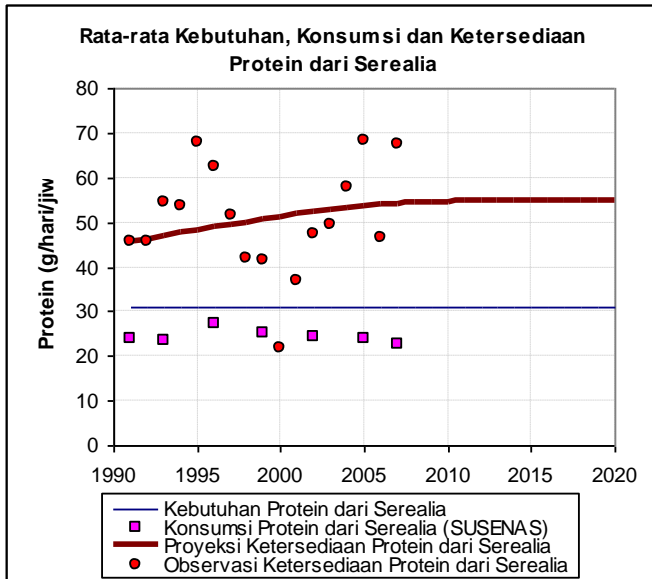
Gambar 14. Rata-rata kebutuhan, konsumsi dan ketersediaan protein perkapita dari serealia di Kabupaten Aceh Selatan tahun 1991-2020.
