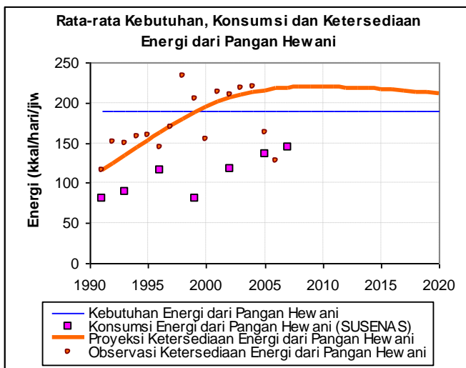
Gambar 12. Rata-rata kebutuhan, konsumsi, dan ketersediaan energi perkapita dari pangan hewani di Kabupaten Aceh Selatan tahun 1991-2020.
