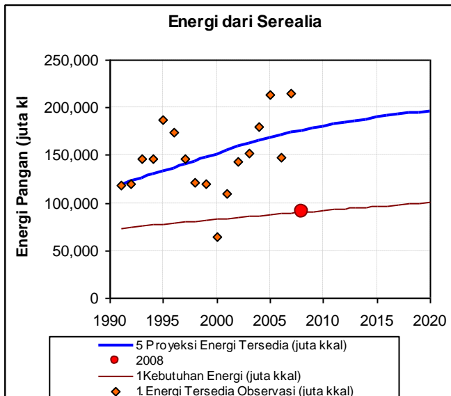
Gambar 9. Proyeksi kebutuhan dan ketersediaan energi pangan dari sereal Kabupaten Aceh Selatan tahun 1991-2020.
