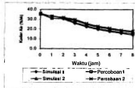
Gambar 7. Hubungan antara waktu dan kadar air gabah dalam tumpukan pada ketebalan 2-3 cm
