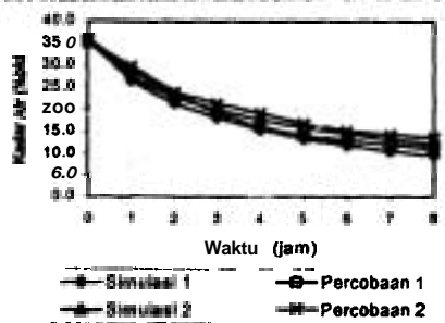
Gambar 6. Hubungan antara waktu dan kadar air gabah dalam tumpukan atas (0-1 cm)
