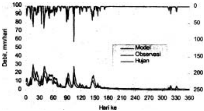
Gambar 6. Grafik Hasil Validasi Data Tahun 1997
