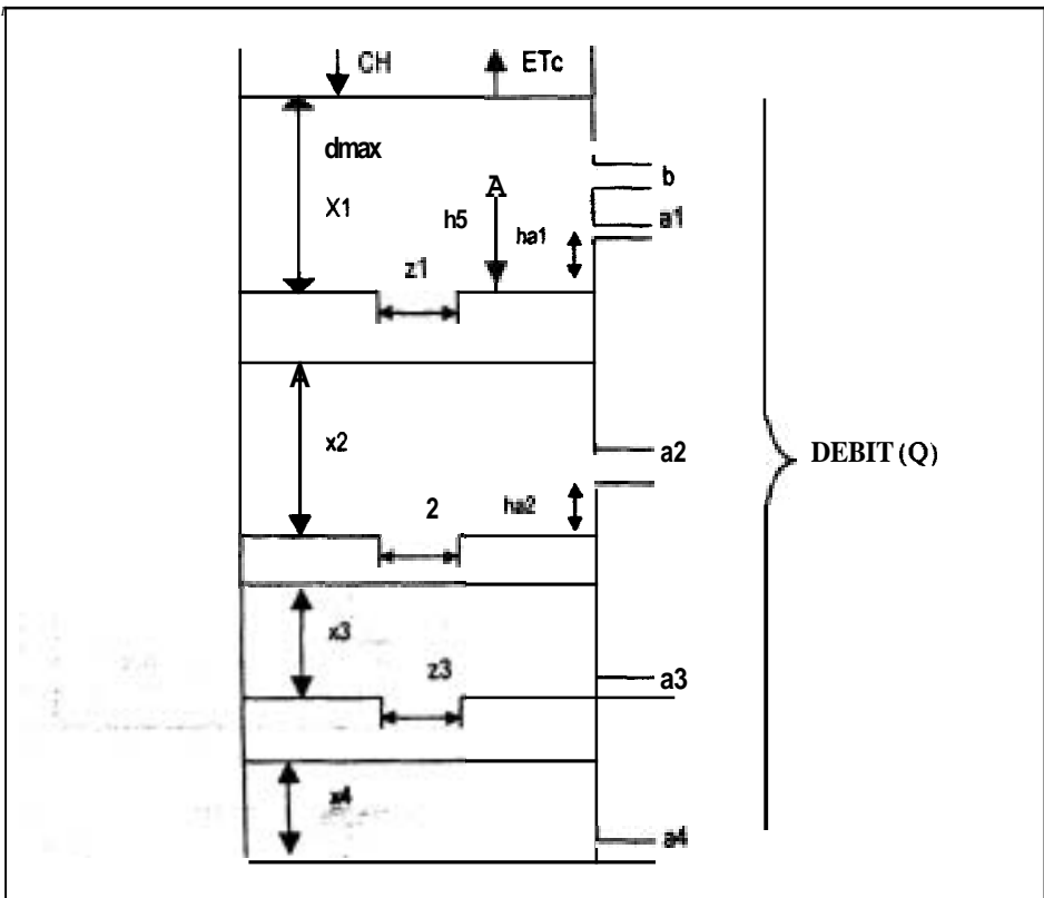
Gambar 2. Skema Tangki untuk Setiap TGL pada Sub DAS
