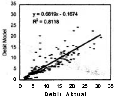
Gambar 7. Hubungan Antara Debit Aktual dan Debit Model Data Tahun 1997
