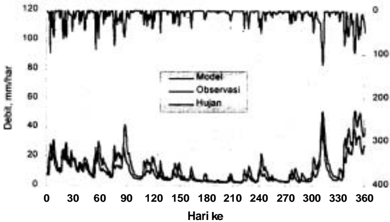
Gambar 4. Grafik Hasil Kalibrasi Data Tahun 1996
