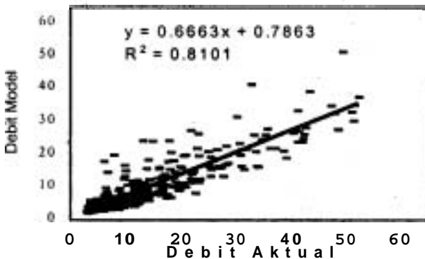
Gambar 5. Hubungan Antara Debit Aktual dan Debit Model Data Tahun 1996
