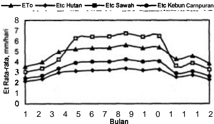
Gambar 3. Rata-Rata Bulanan Evapotranspirasi Tahun 1996
