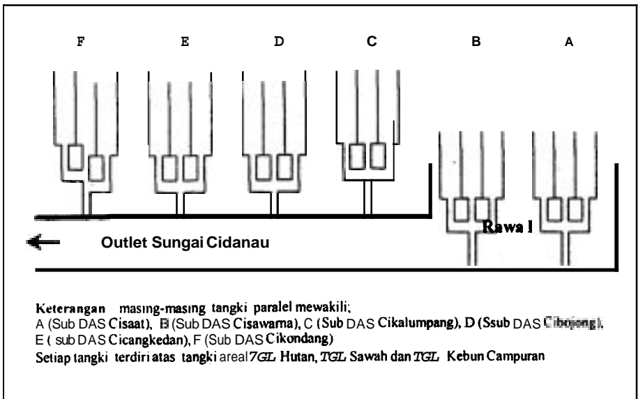
Gambar 1. Susunan Tangki untuk DAS Cidanau
