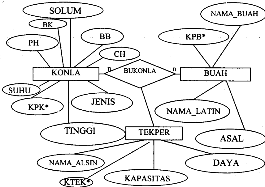
Gambar 1. ERD yang Mendeskripsikan Relasi antara Entiti Tanaman Buah-buahan dan Entiti Kondisi Agroklimat Lahan
