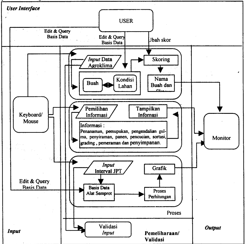
Gambar 3. Arsitektur Sistem
