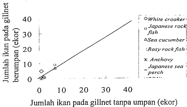
Gambar 4. Perbandingan jumlah tangkapan antara gillnet yang dipasang umpan dan tanpa umpan.
