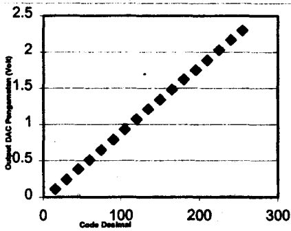
Gambar 5. Hubungan set desimal dan tegangan Keluaran DAC
