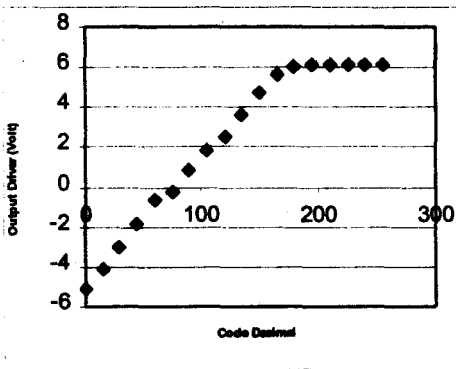
Gambar 6. Hubungan antara set desimal dan tegangan
