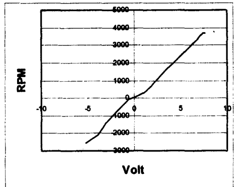
Gambar 7. Grafik tegangan kerja versus rpm motor pada pencatuan 9 Volt
