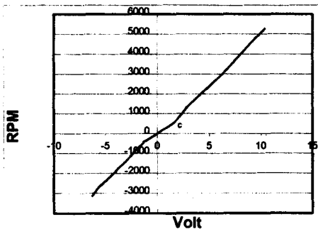
Gambar 8. Grafik hubungan tegangan kerja dan rpm motor pada pencatuan 12 Volt
