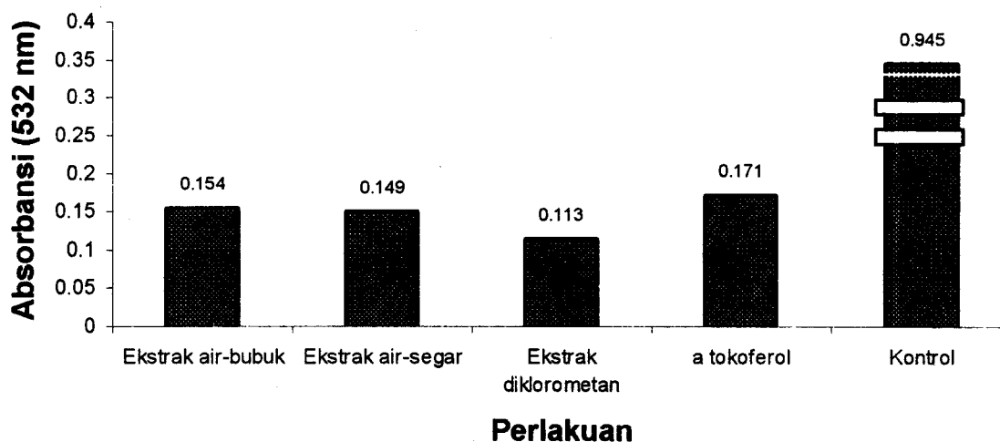
Gambar 3. Absorbans malonaldehid dari asam linoleat yang disuplementasi ekstrak jahe dan inkubasi selama 16 hari.
