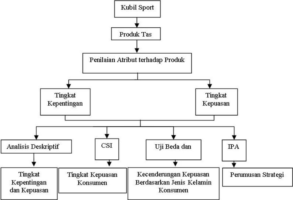
Gambar 1. Kerangka Pemikiran
